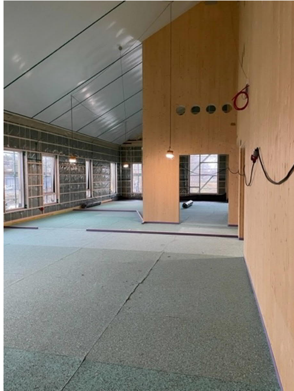
Isoleringskiva (stepisol) utlagd på träbjälklaget inför flytspackling på plan 2 Hus 2.
